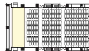
3 ■ テルサホール.03 スラストステージタイプ
