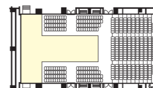
5 ■ テルサホール.05 フルフラット&アトリウムチャラー一体型タイプ
